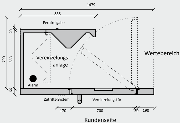
Grundriss
