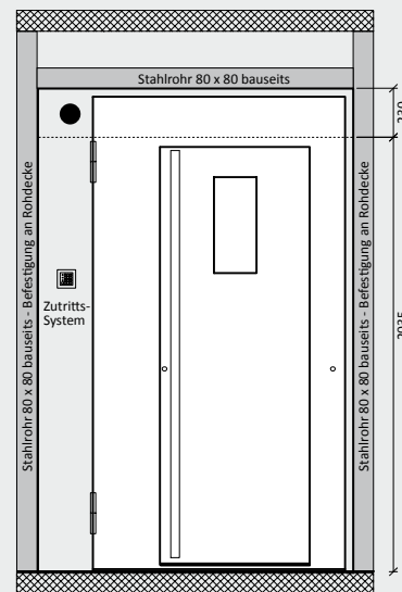
Ansicht Kundenseite
